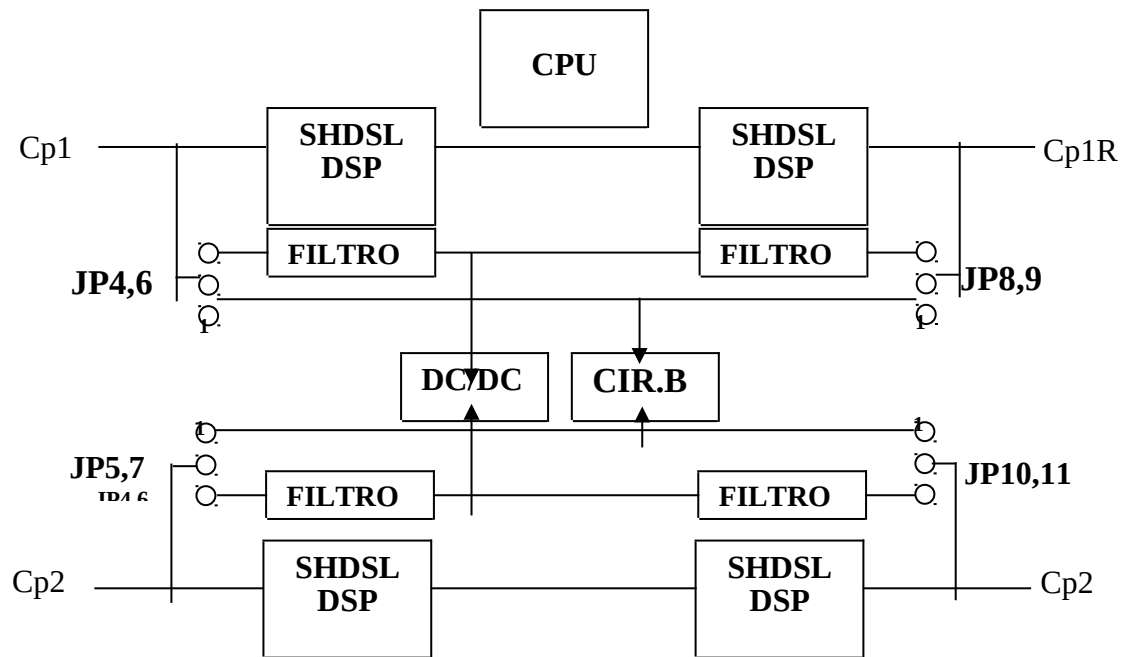
Figura 3: schema a blocchi del rigeneratore
